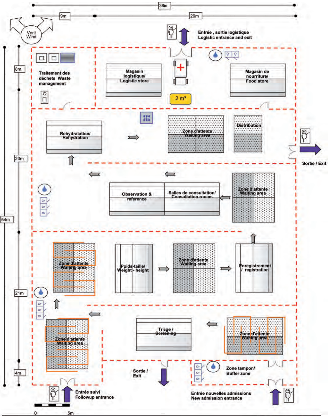
Centre de nutrition supplémentaire (circuit ration sèche) Supplementary feeding centre (dry ration circuit)
