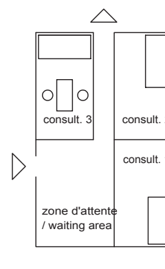
TENTE AVEC 3 SALLES DE CONSULTATION ET ZONE D'ATTENTE / TENT WITH 4 CONSULTATION ROOMS AND WAITING AREA
