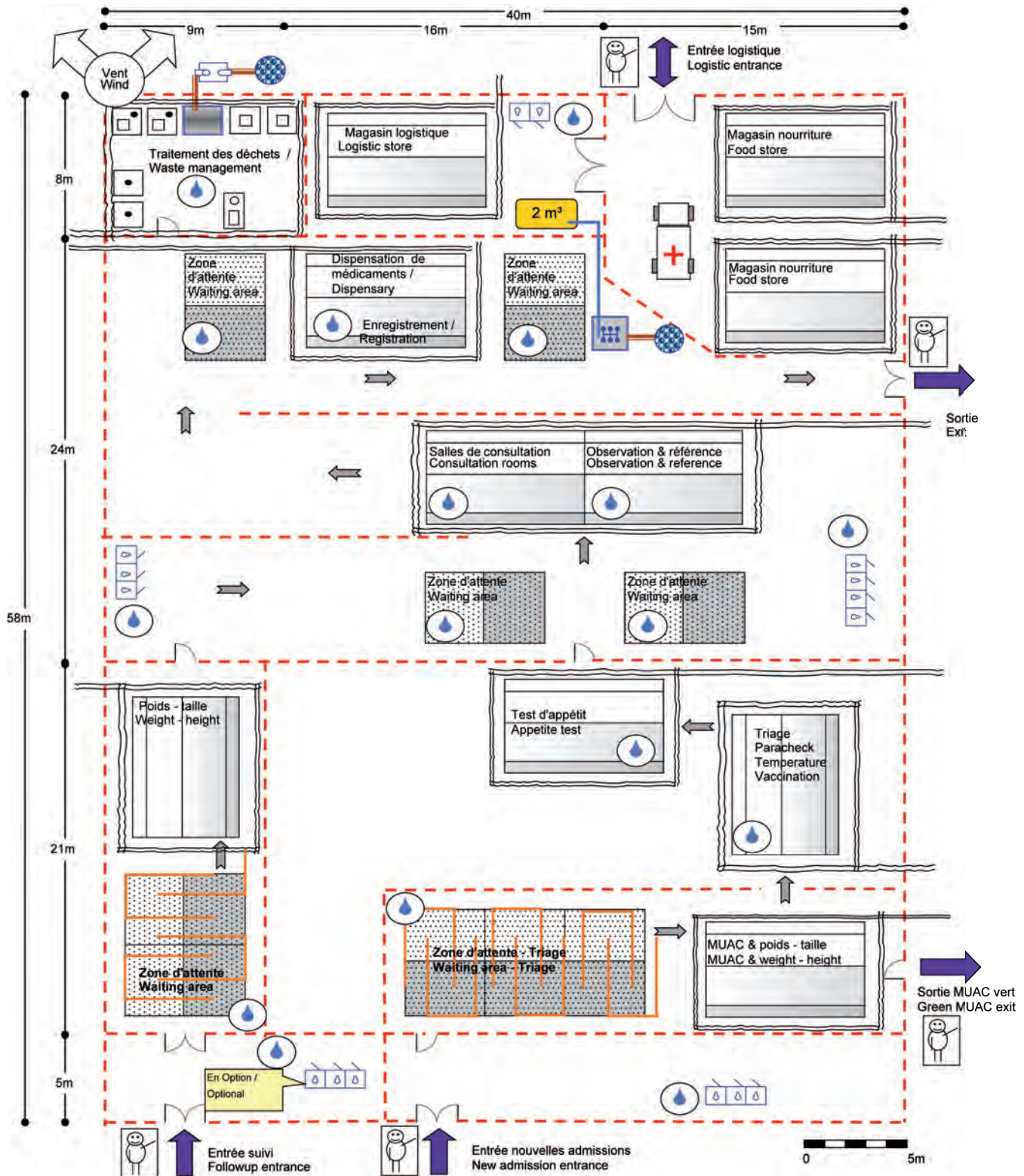
Eau et assainissement / Water and Sanitation Centre de nutrition thérapeutique ambulatoire Ambulatory therapeutic feeding centre Capacité : 150 bénéf./jour Capacity: 150 benef./day 15m 2 / benef.
